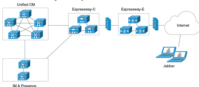
图 4: 客户端连接到 Expressway for Mobile and Remote Access 的方式
