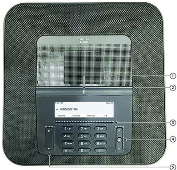
Figura 2: Botones y funciones del Teléfono IP para conferencias Cisco 8832
