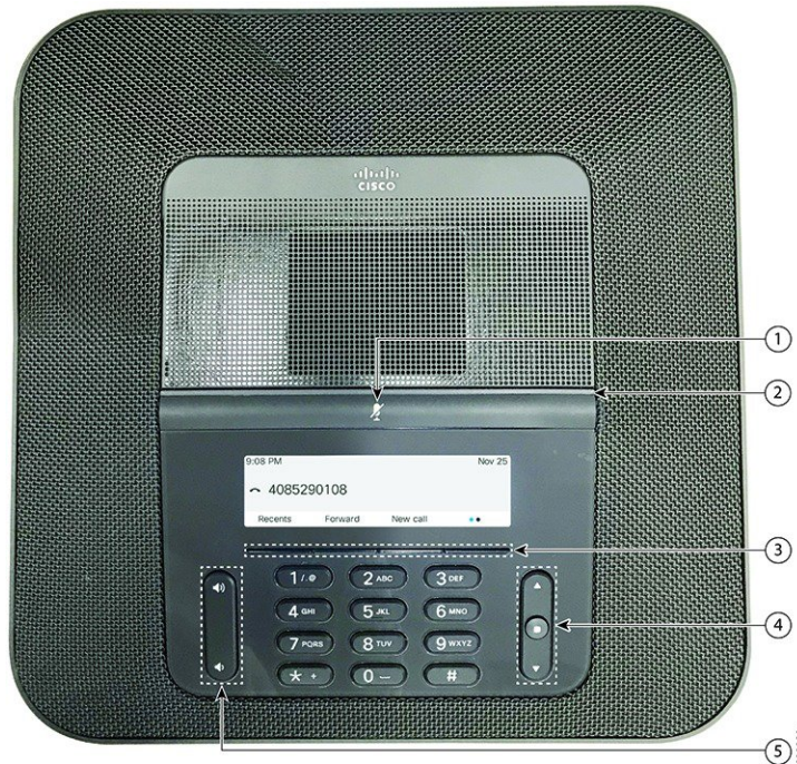
图 2: Cisco IP Conference Phone 8832 按键和功能
