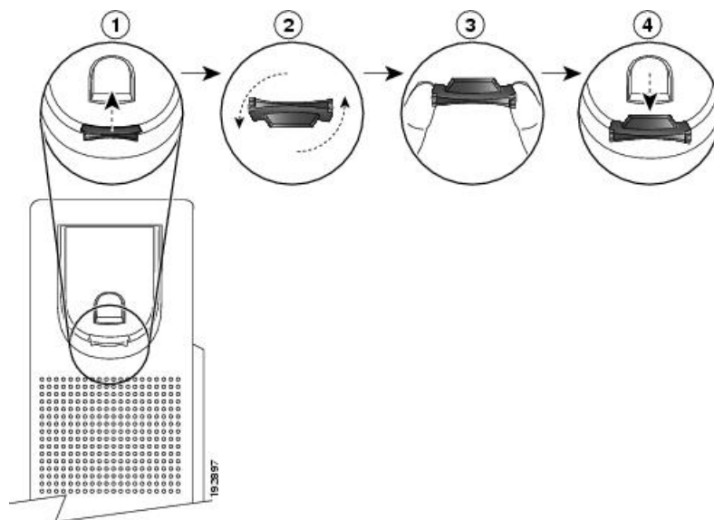
Figur 16: Juster håndsætholderen
