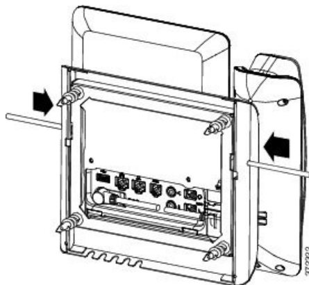
Figur 15: Frakobl tapperne
