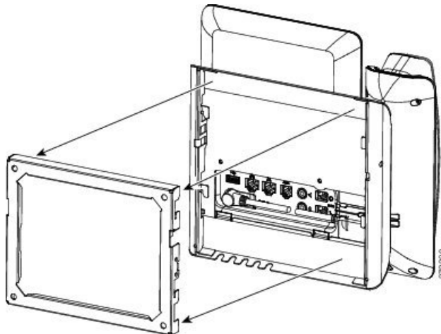
Figur 13: Fastgør telefonen til vægbeslaget
