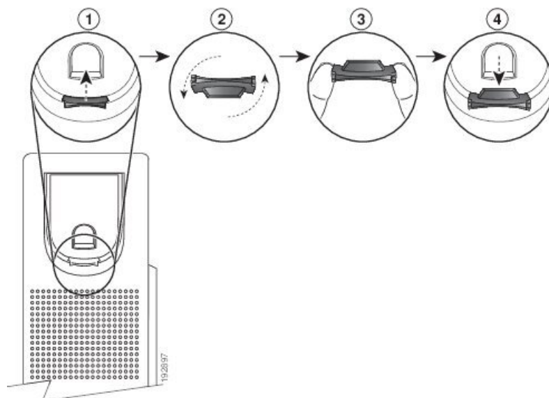
图题 26: 調整聽筒座
