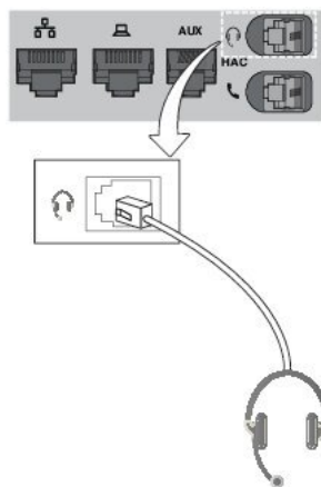
图题 19: 連接標準耳機
