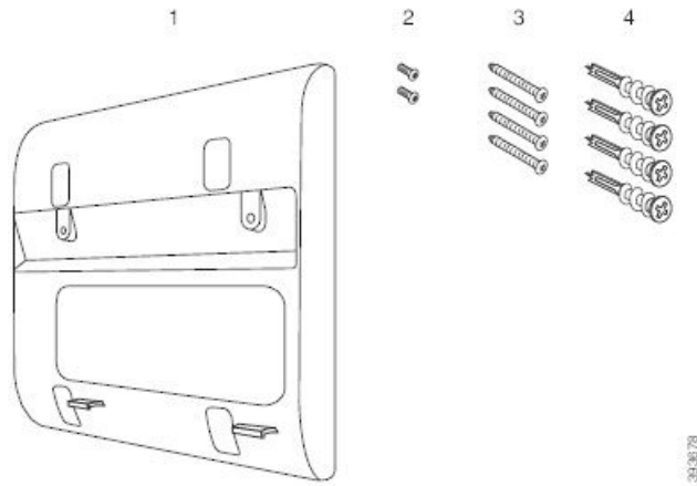
图題 20: Cisco IP 電話 6800 系列多平台電話掛牆式安裝套件
