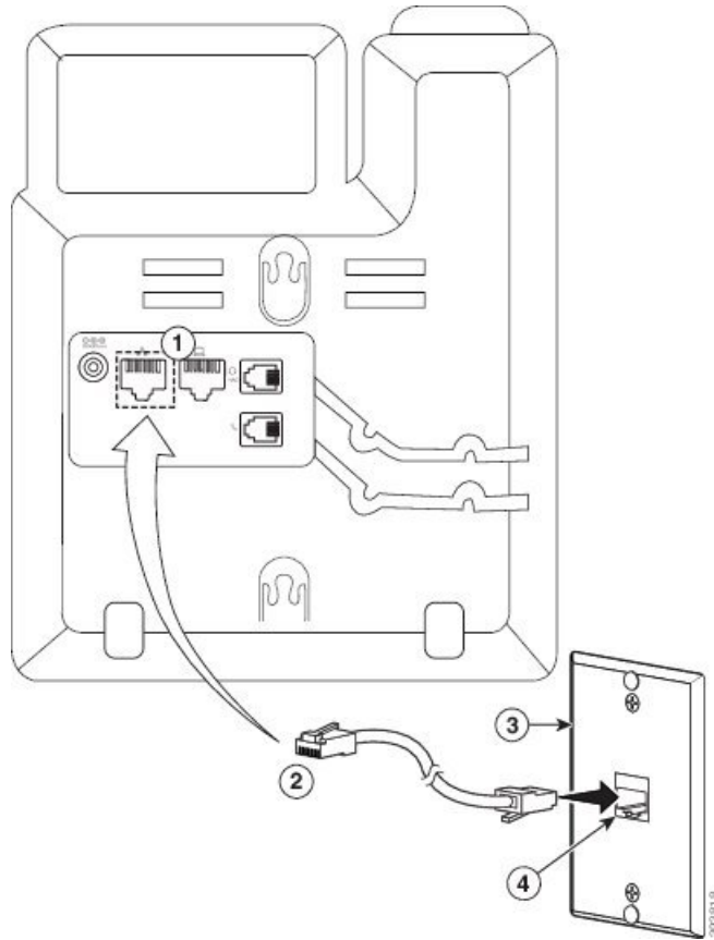
图题 23: 掛牆安裝板插孔中的 RJ45 連線器
