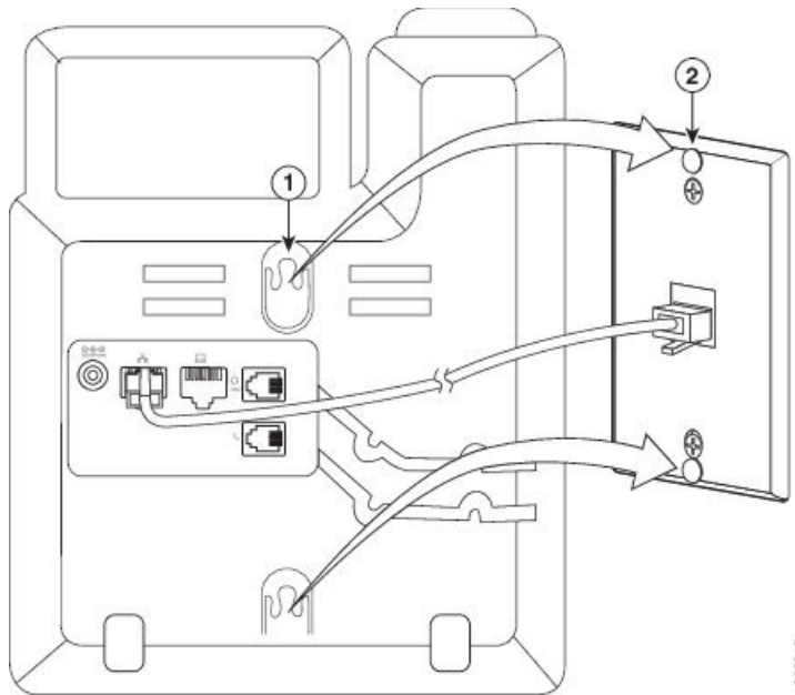
圖題 24: 固定孔
