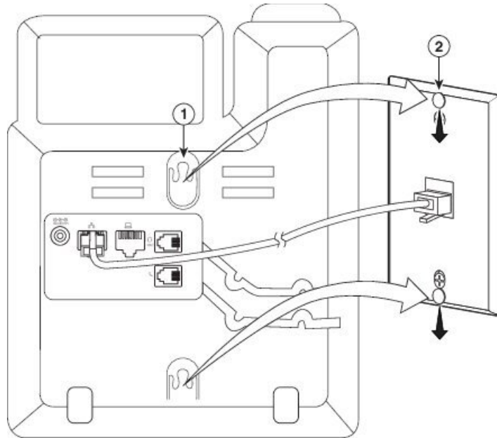
图题 25: 套緊 IP 電話
