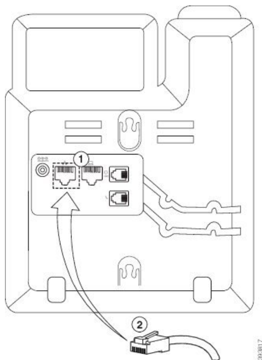
图题 22: 電話插孔的 RJ45 連線器
