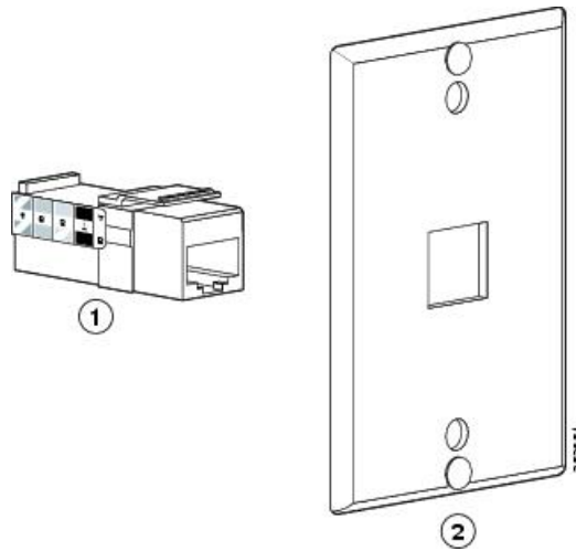
Figura 10: Placa de montaje de pared Leviton
