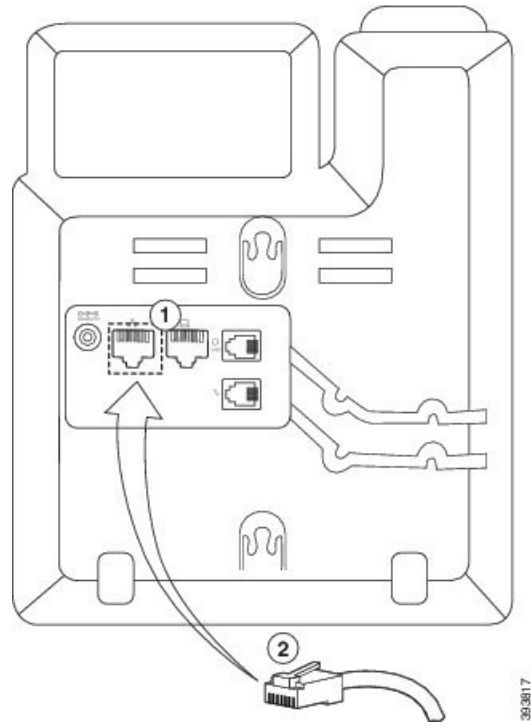
Figura 11: Conector RJ45 en el conector del teléfono
