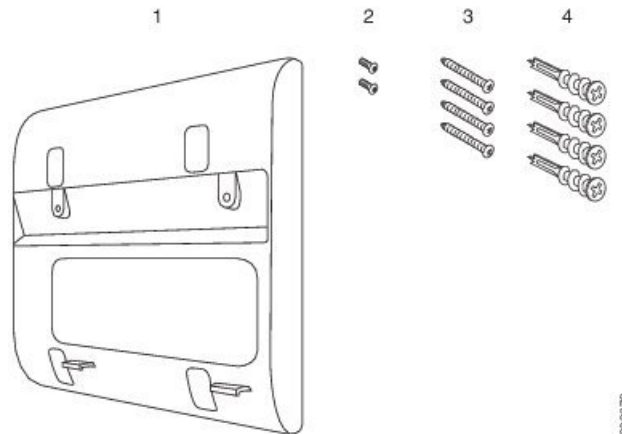
Figura 9: Kit de montaje de pared de los teléfonos multiplataforma IP Cisco serie 6800
