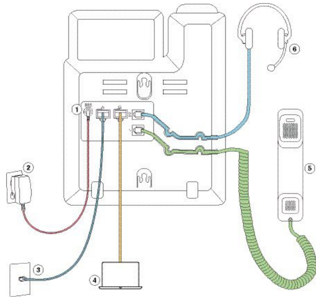
Figura 2: Teléfonos multiplataforma IP Cisco 6821 Conexiones
