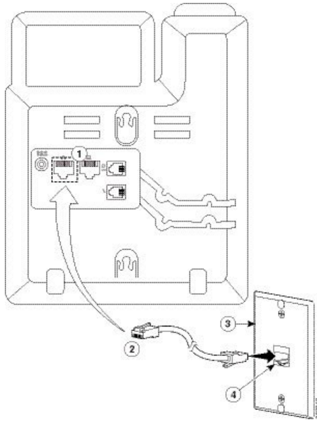
Figura 12: Conector RJ45 en el conector de montaje de pared
