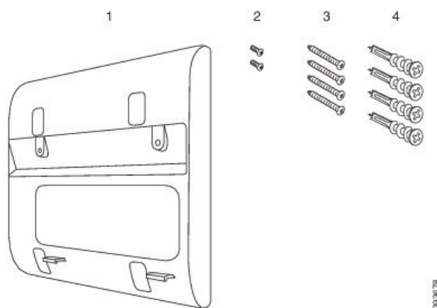
Figura 5: Kit di montaggio a parete dei telefoni multiplatforma Cisco IP Phone serie 6800
