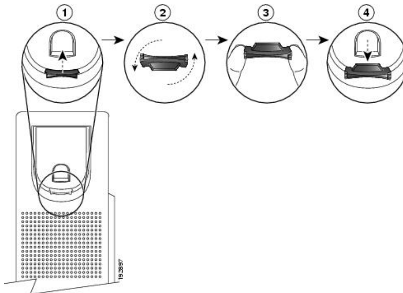
Figura 11: Regolazione del supporto del ricevitore
