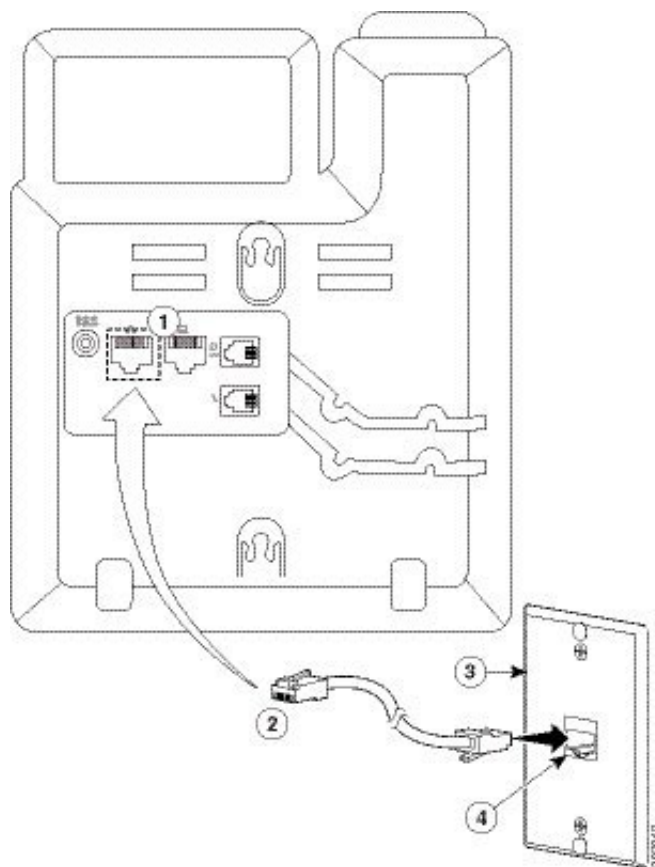
Figura 8: Connettore RJ45 nella presa di montaggio a parete
