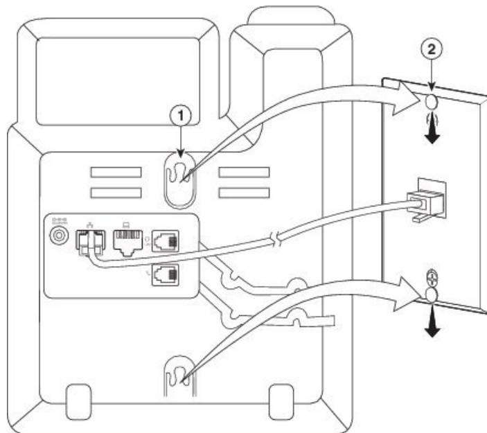
Figura 10: Scorrimento del telefono IP
