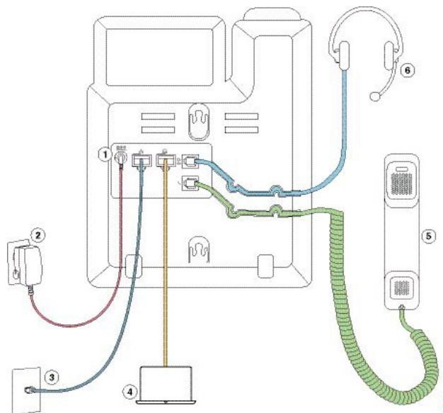
Figura 2: Collegamenti dei Telefoni multiplatforma Cisco IP Phone 6821
