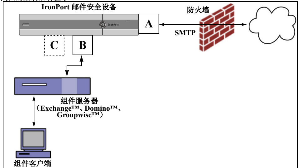
图 40-4 企业网关的黑洞侦听程序
