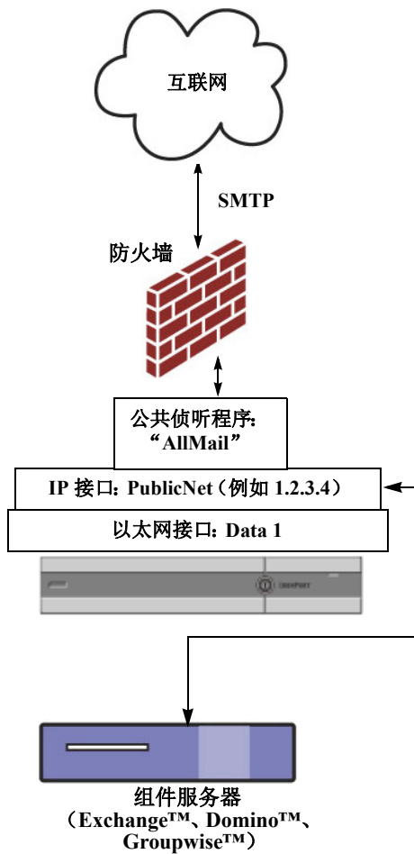
图 3-2 一个侦听程序配置
