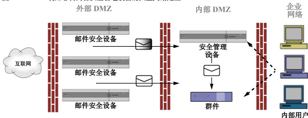
图 42-1 利用思科内容安全管理设备的典型网络配置
