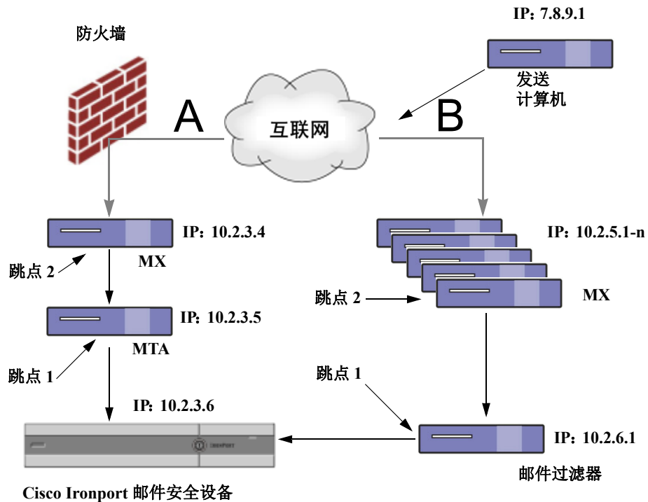
图 13-5 通过 MX/MTA 中继的邮件 - 高级
