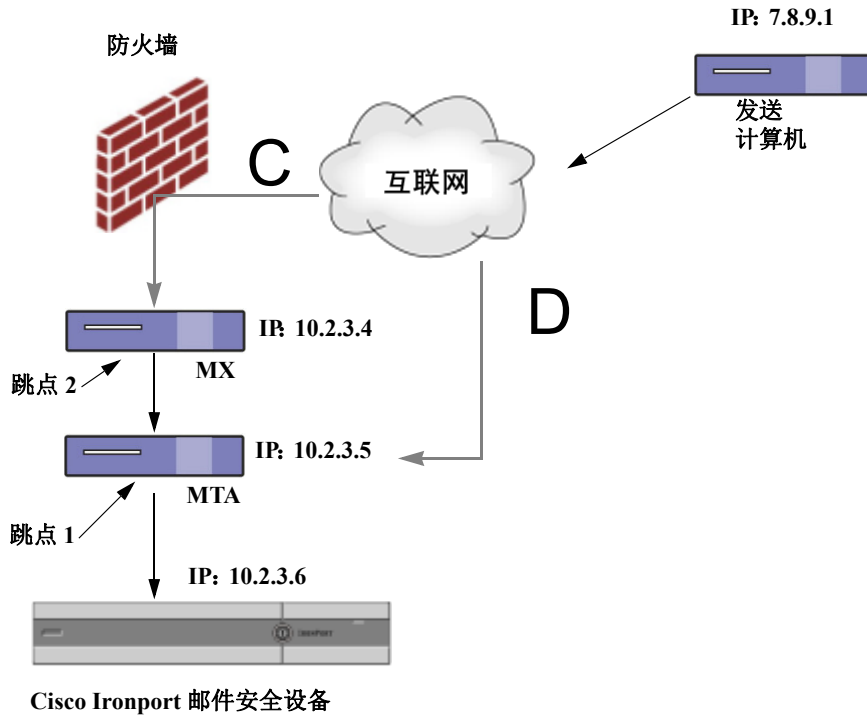
图 13-6 MX/MTA 中继的邮件 - 可变跳数
