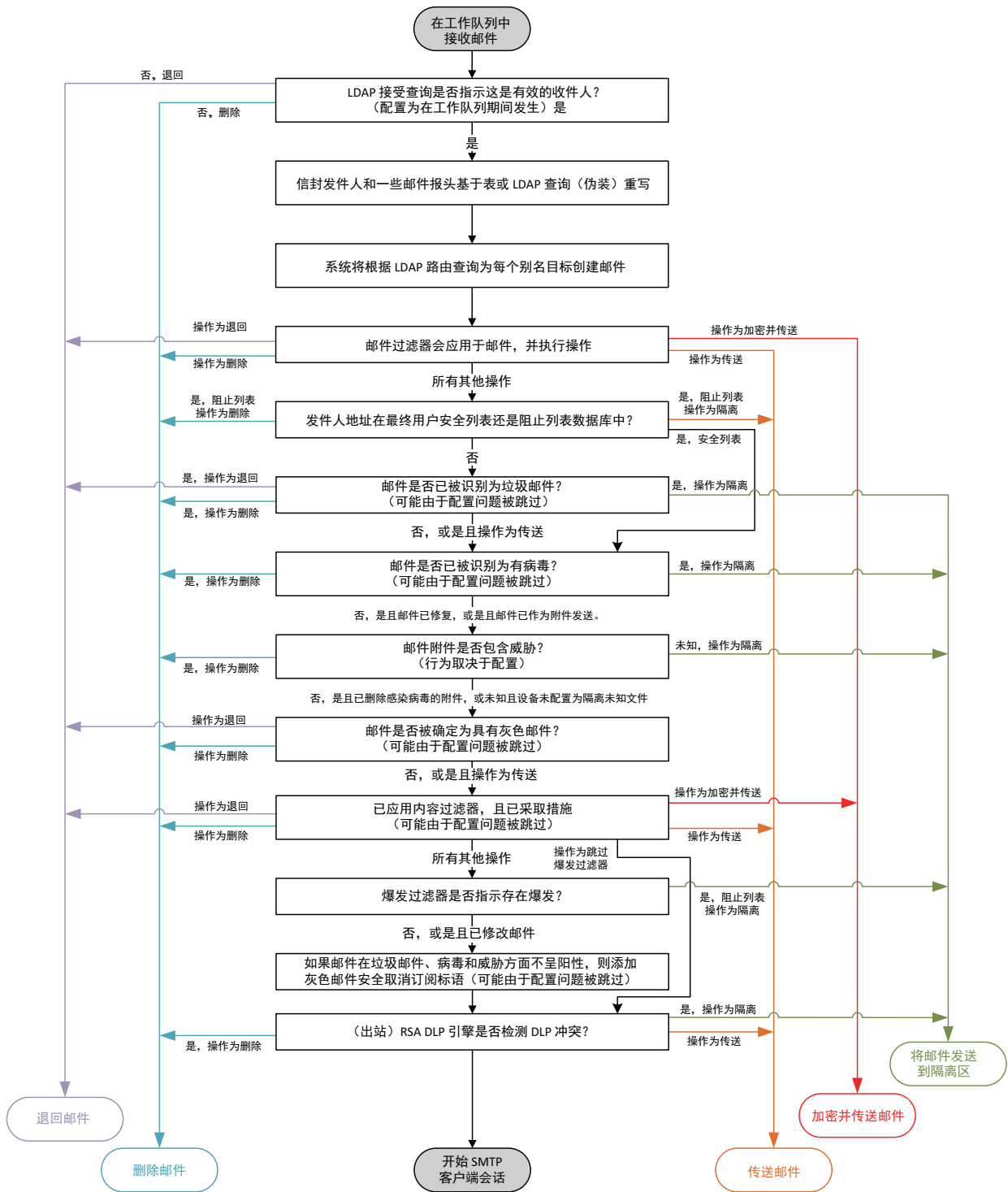
图 4-2 邮件管道 - 工作队列
