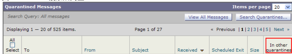
图 30-2 搜索隔离区
