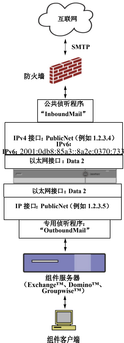
图 3-1 防火墙保护的场景 / 2 个侦听程序配置
