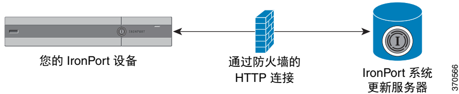
图 33-1 流更新方法
