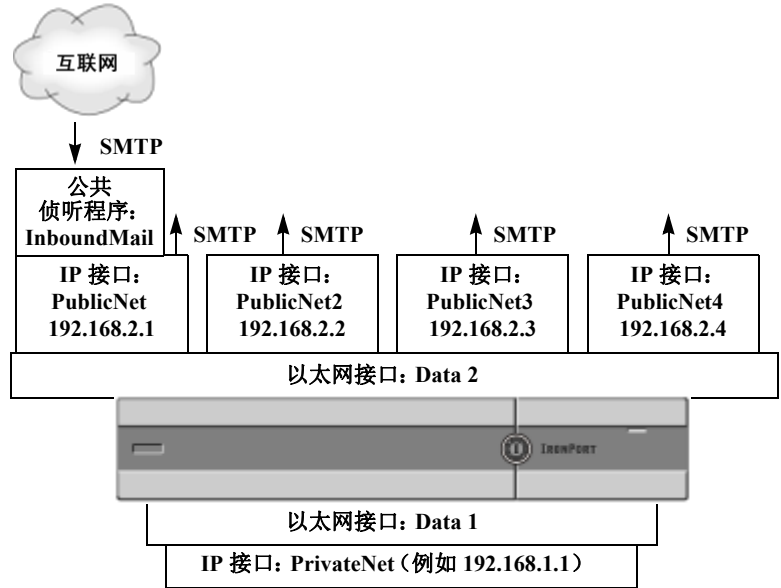
图 25-13 在一个以太网接口上配置四个虚拟网关地址
