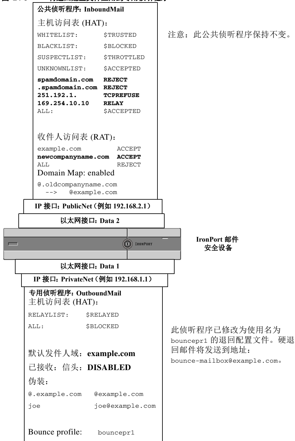
图 24-5 将退回配置文件应用到专用侦听程序
