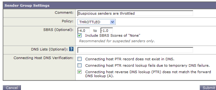
图 7-6 发件人组: SUSPECTLIST: 编辑设置
