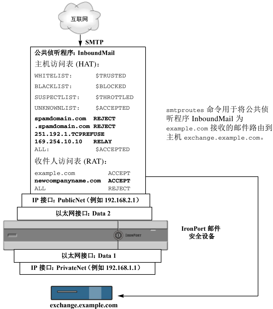
图 24-1 为公共侦听程序定义的 SMTP 路由
