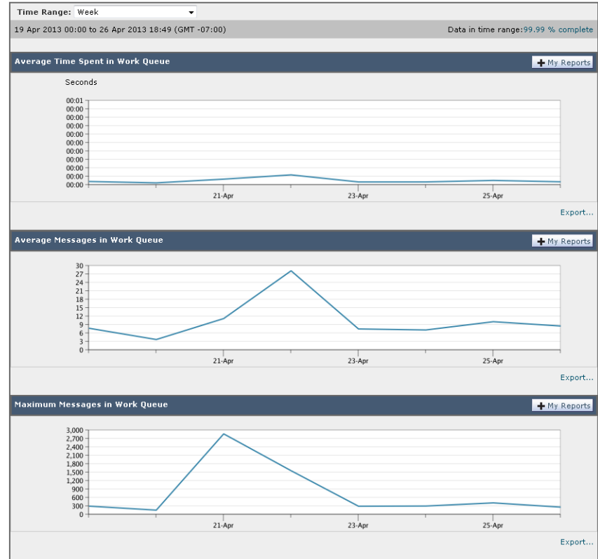
图 28-1 系统容量 - 工作队列 System Capacity
