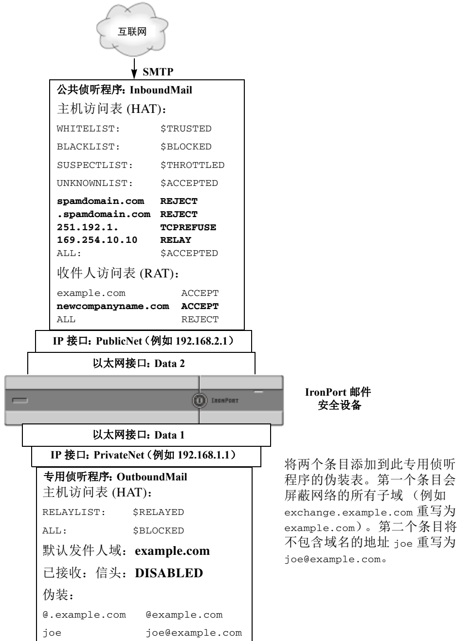
图 24-3 为专用侦听程序定义的伪装
