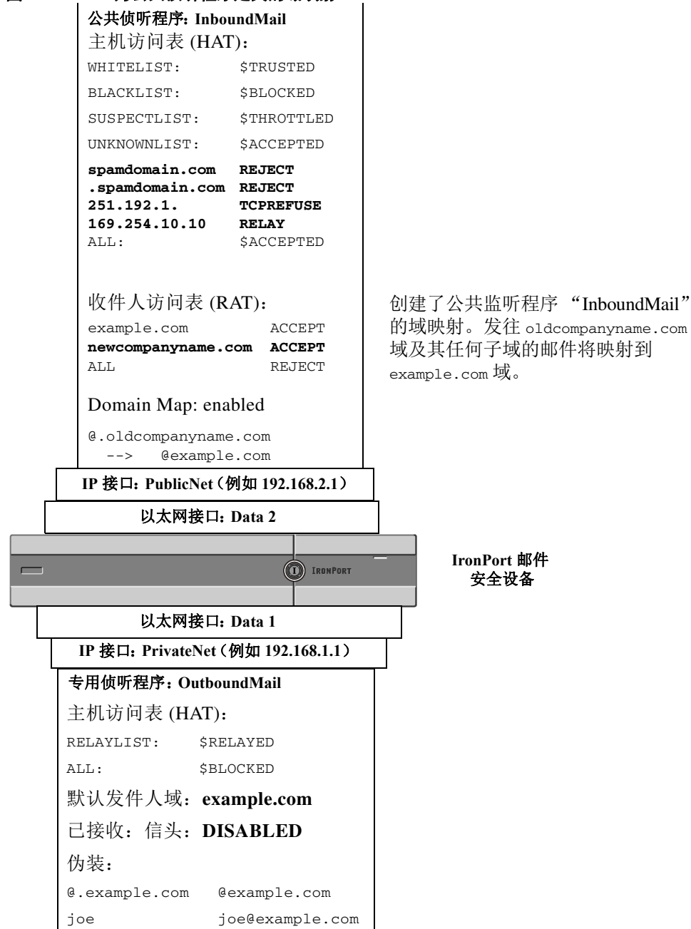
图 24-4 为公共侦听程序定义的域映射
