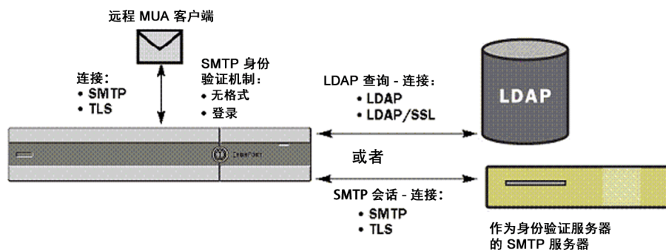
图 25-11 SMTP Auth 支持：LDAP 目录存储或 SMTP 服务器
