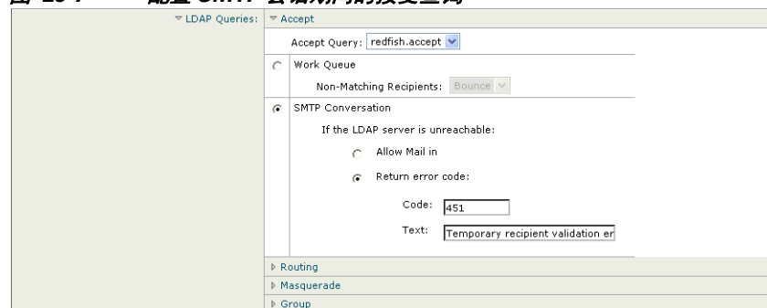
图 25-7 配置 SMTP 会话期间的接受查询
