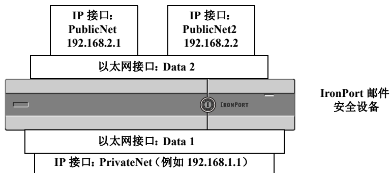
图 24-10 添加另一个公共接口
