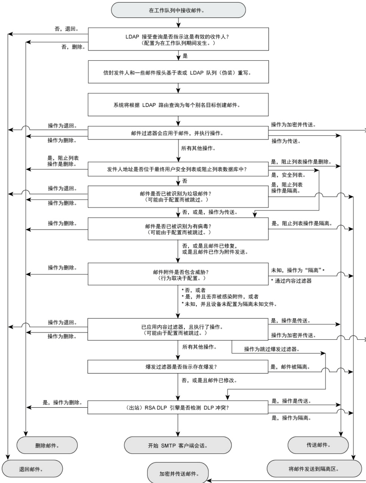
图 4-2 邮件管道 - 工作队列
