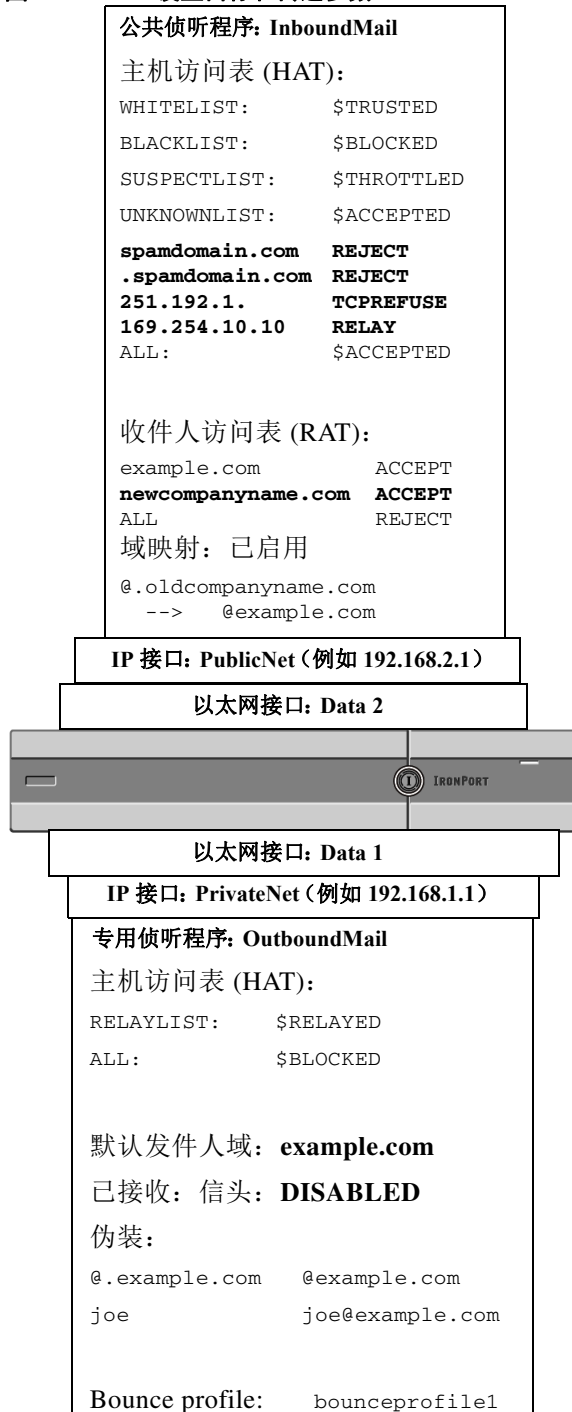
图 24-8 设置目标和传送参数
