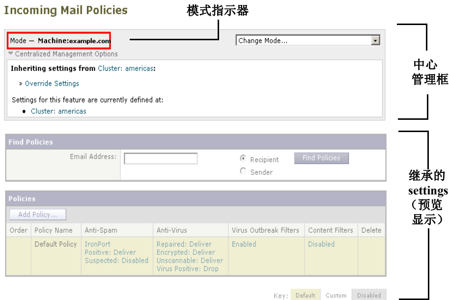
图 39-2 GUI 中的集中管理功能：未定义设置
