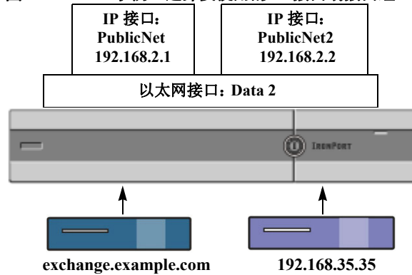
图 24-12 示例：选择要使用的 IP 接口或接口组
