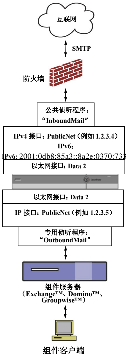
图 3-1 防火墙保护的场景/2 个侦听程序配置
