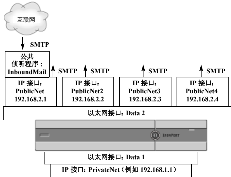
图 24-11 在一个以太网接口上配置四个虚拟网关地址
