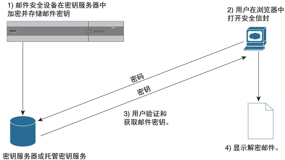
图 18-1 加密工作流程
