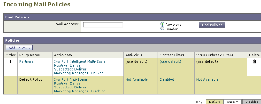
图 13-3 邮件策略 - 在策略中启用智能多扫描
