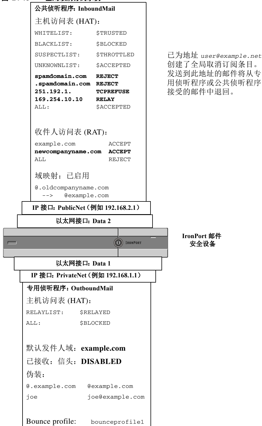
图 24-13 全局取消订阅示例
