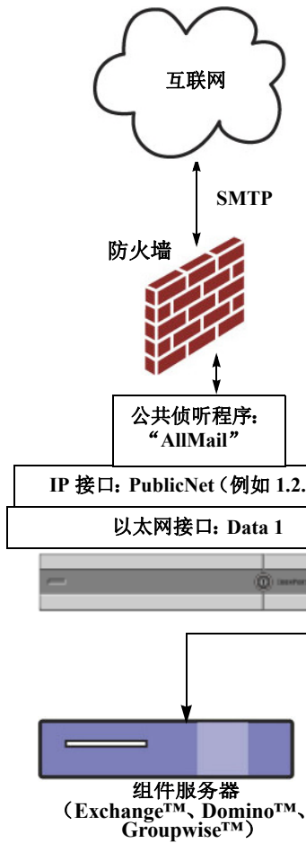
图 3-2 一个侦听程序配置
