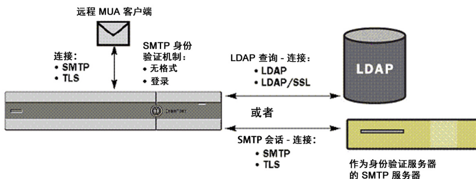
图 25-11 SMTP Auth 支持：LDAP 目录存储或 SMTP 服务器
