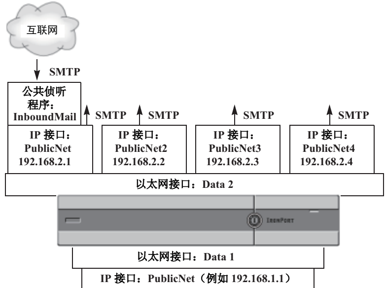
图 24-13 在一个以太网接口上配置四个虚拟网关地址
