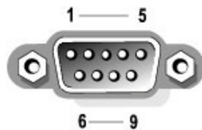
图 A-2 串行端口的引脚编号
