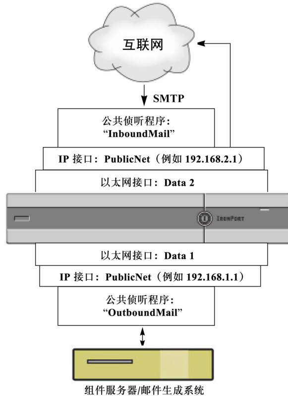
图 5-2 具有两个以上以太网接口的设备型号上的公共和专用侦听程序
