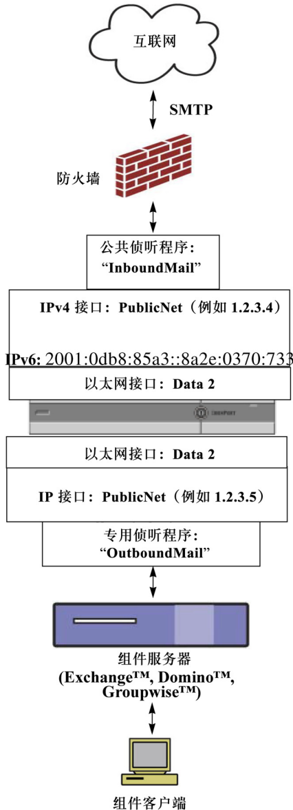
图 3-1 防火墙后情景/双侦听程序配置
