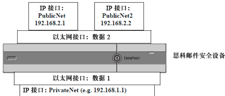
图 26-10 添加另一个公共接口
