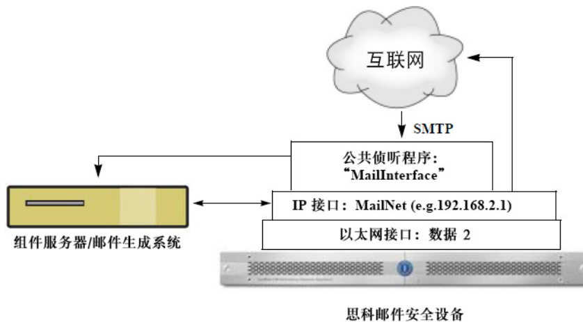
图 5-3 多种型号仅有两个以太网接口的设备上的公共侦听程序
