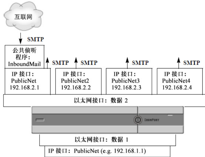
图 26-11 在一个以太网接口上配置四个虚拟网关地址
