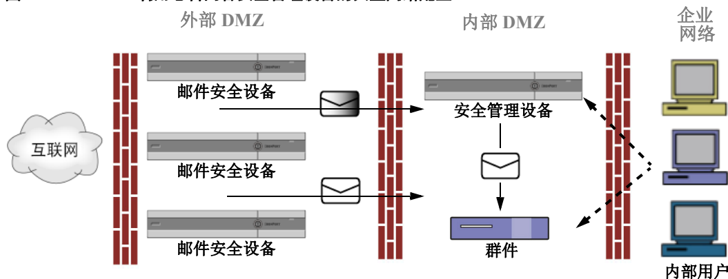
图 43-1 利用思科内容安全管理设备的典型网络配置
