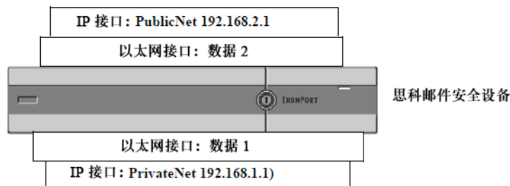
图 26-7 公共和专用接口示例
