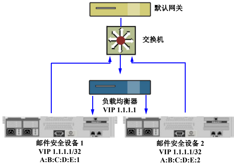
图 38-2 使用 DSR 实现交换机上多个邮件安全设备之间的负载均衡
