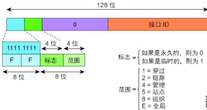
图 77: IPv6 组播地址格式
