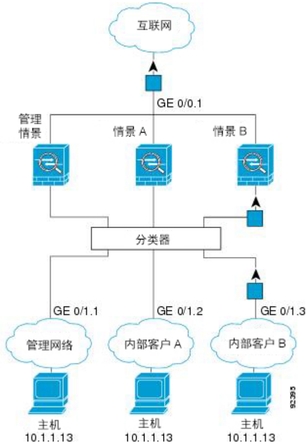
图 32: 来自内部网络的传入流量
