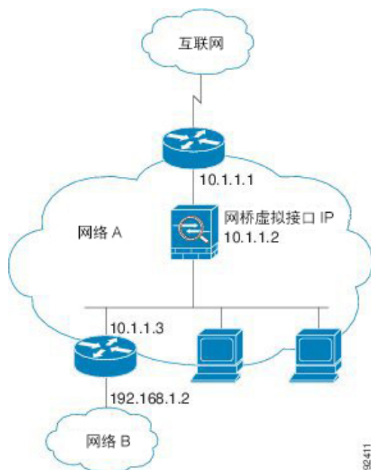
图 17: 透明防火墙网络
