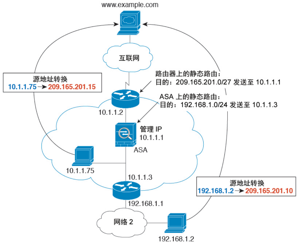
图 20: NAT 示例：网桥组中的 NAT
