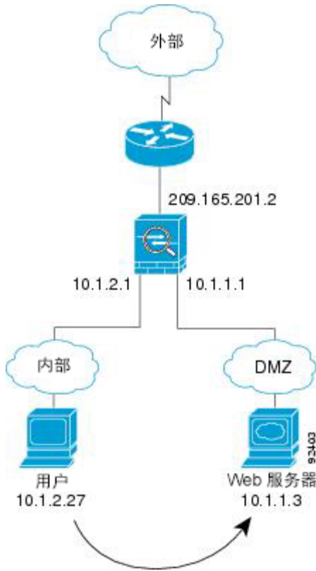
图 23: 从内部到 DMZ
