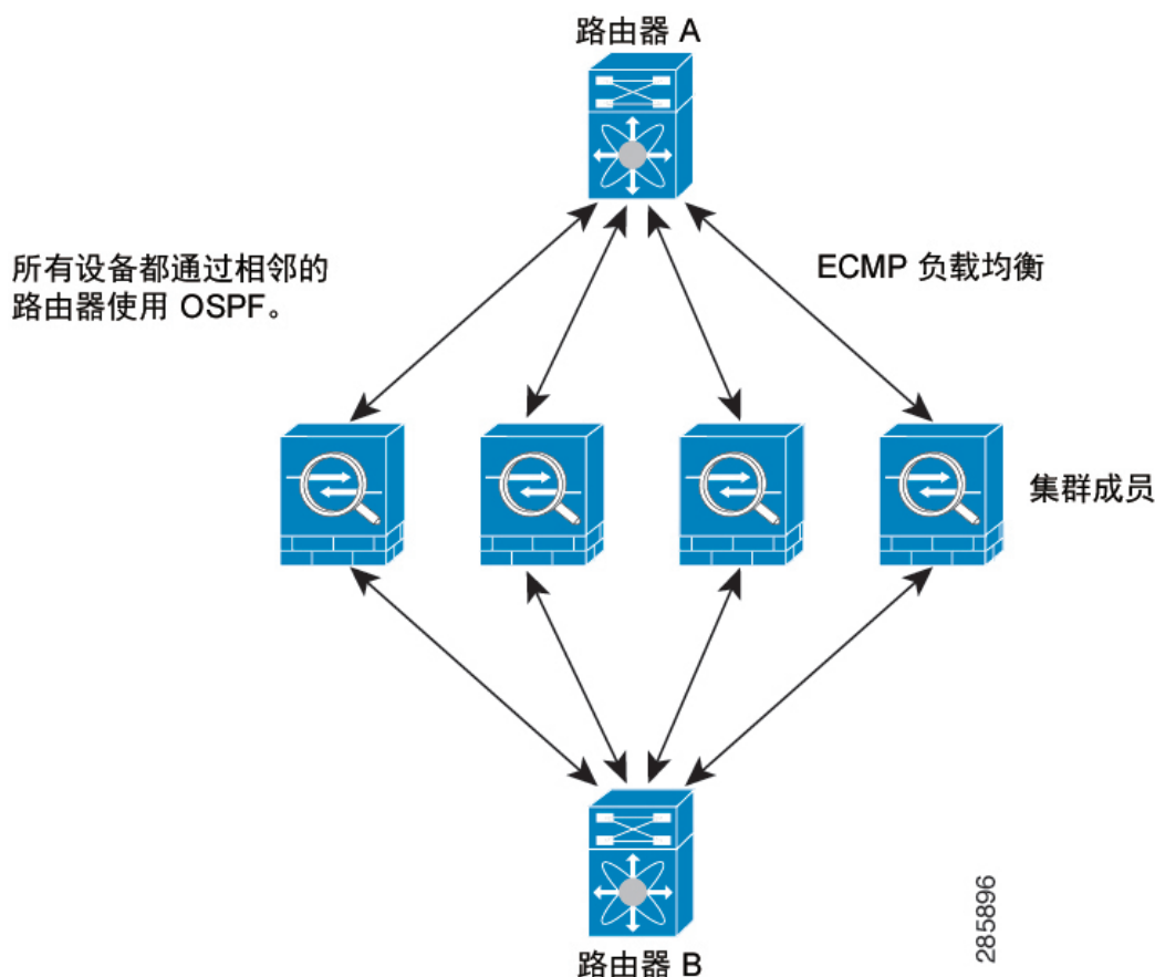
图 60: 独立接口模式下的动态路由
