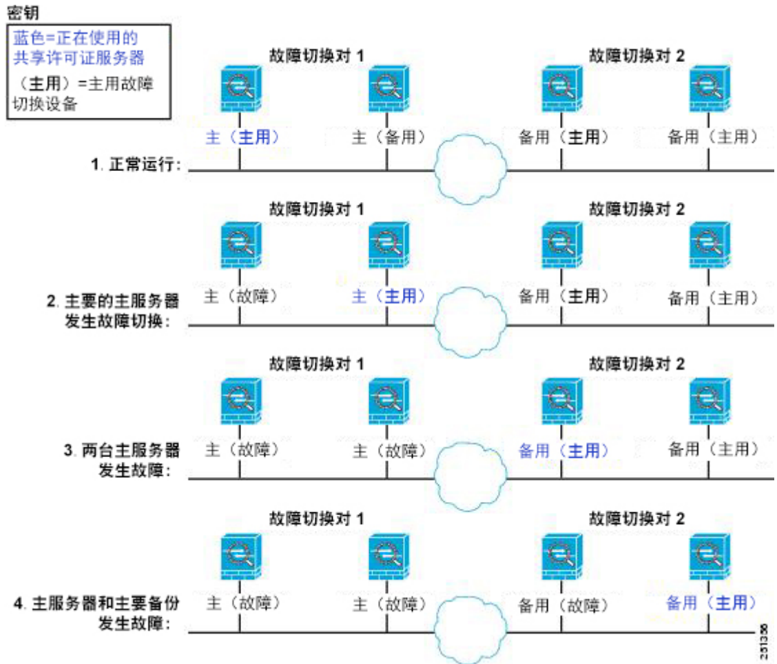
图 6: 故障切换和共享许可证服务器
