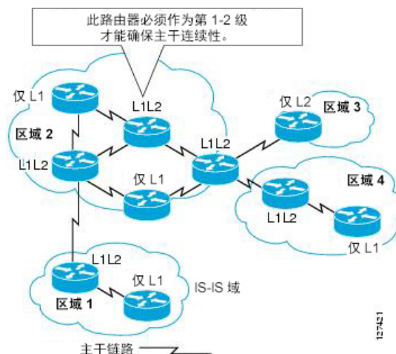
图 64: IS-IS 网络拓扑中的级别 1、级别 2、级别 1-2 设备
