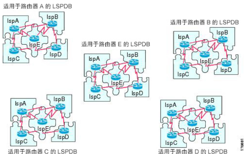
图 66: 包含已同步的 LSPDB 的 IS-IS 设备
