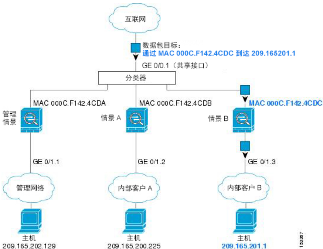
图 31: 使用 MAC 地址通过共享接口进行数据包分类
