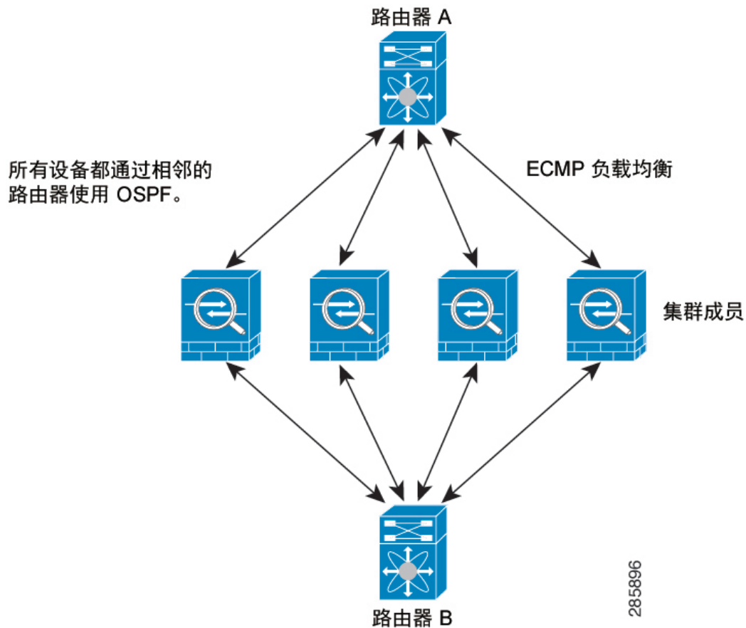
图 53: 独立接口模式下的动态路由
