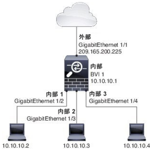
图 19: 具有内部网桥组和外部路由接口的路由防火墙网络
