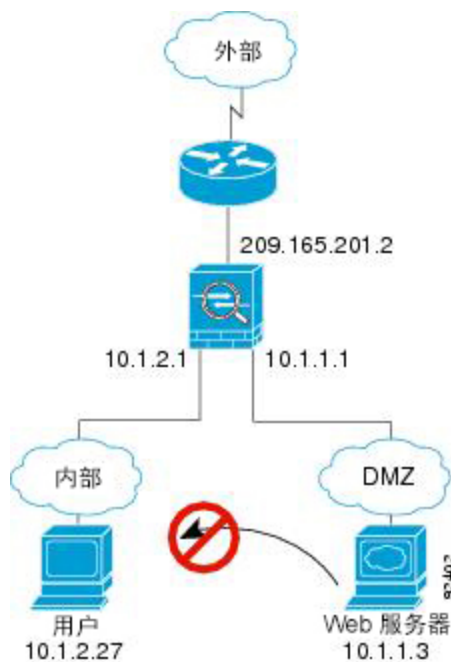
图 25: 从 DMZ 到内部
