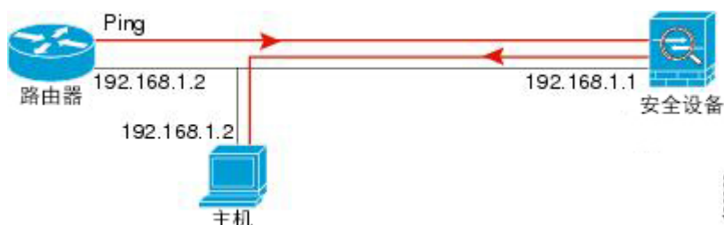
图 74: IP 寻址问题引发的 ping 故障
