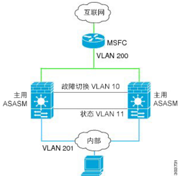
图 49: 网桥组环路
