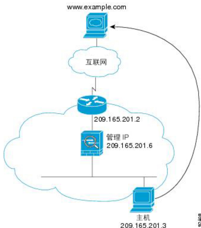
图 27: 内部至外部
