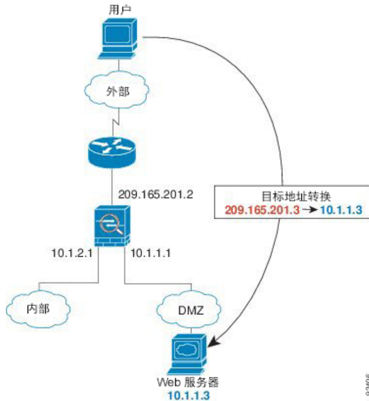
图 22: 外部到 DMZ
