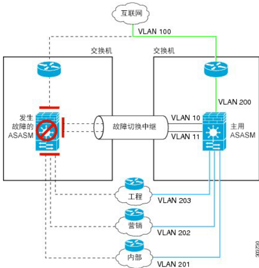
图 47: ASASM 故障
