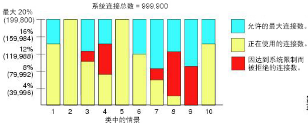
图 36: 资源超订用
