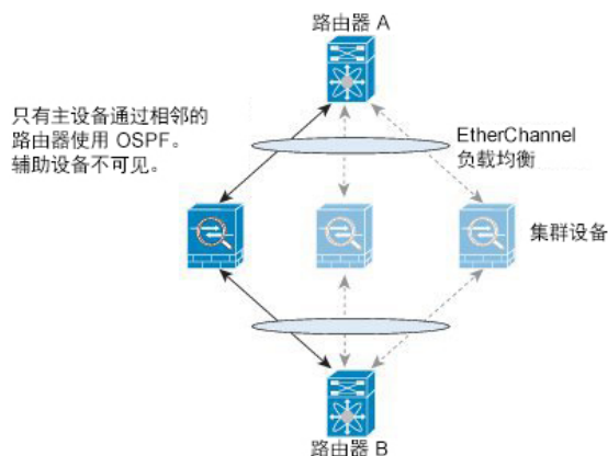
图 54: 动态路由
