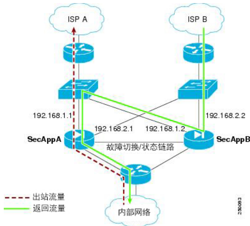
图 50: ASR 示例
