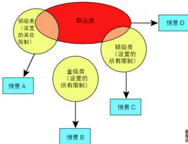
图 35: 资源类
