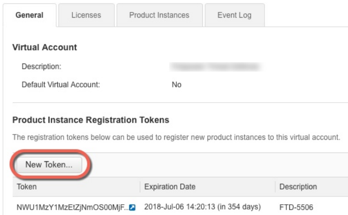
图 8: 新建令牌
