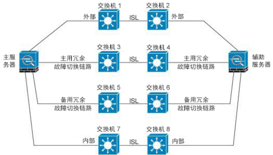
图 44: 使用交换机间链路连接
