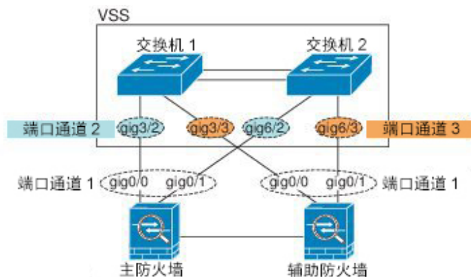
图 56: 主用/备用故障切换和 VSS/vPC
