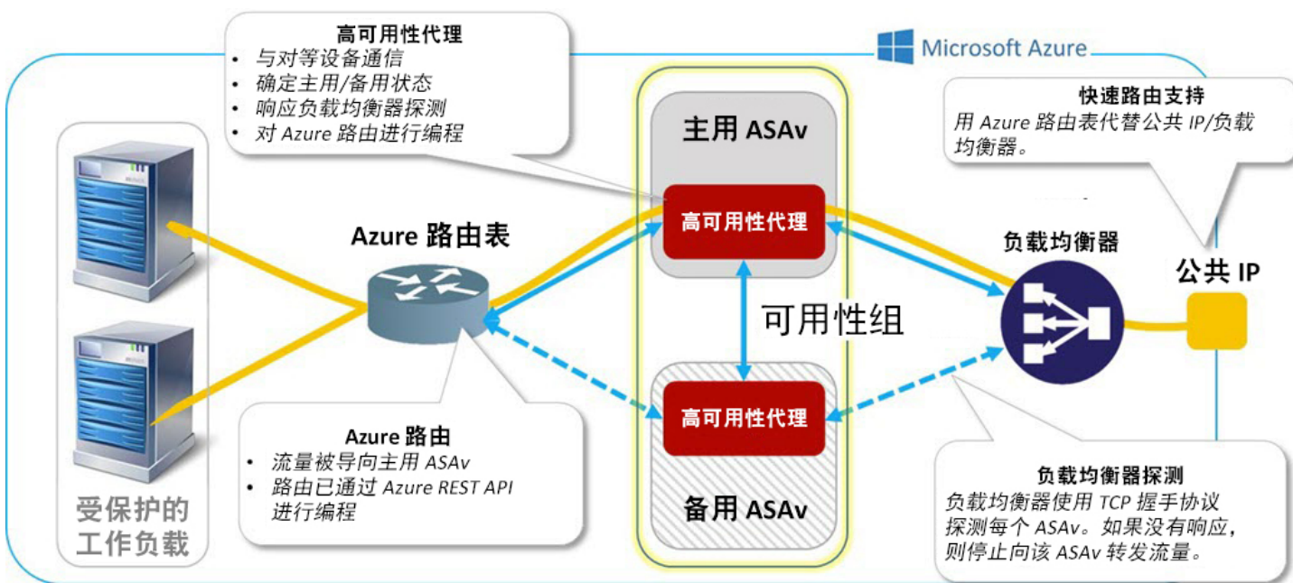
图 51: Azure 中的 ASA HA 部署
