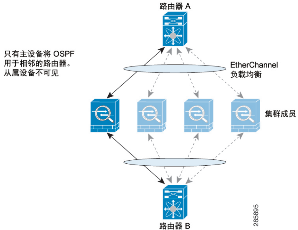
图 52: 跨网络 EtherChannel 模式下的动态路由
