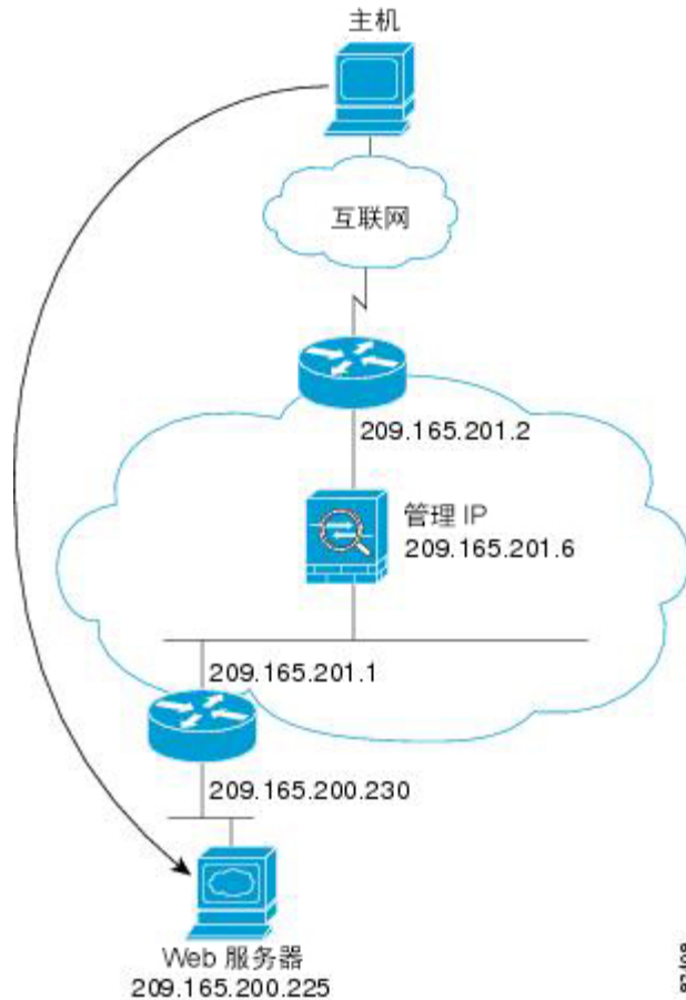
图 29: 从外部到内部
