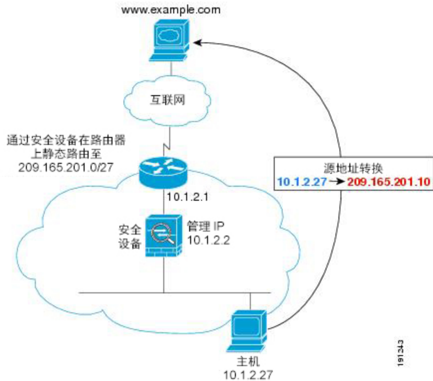
图 28: 使用 NAT 从内部到外部
