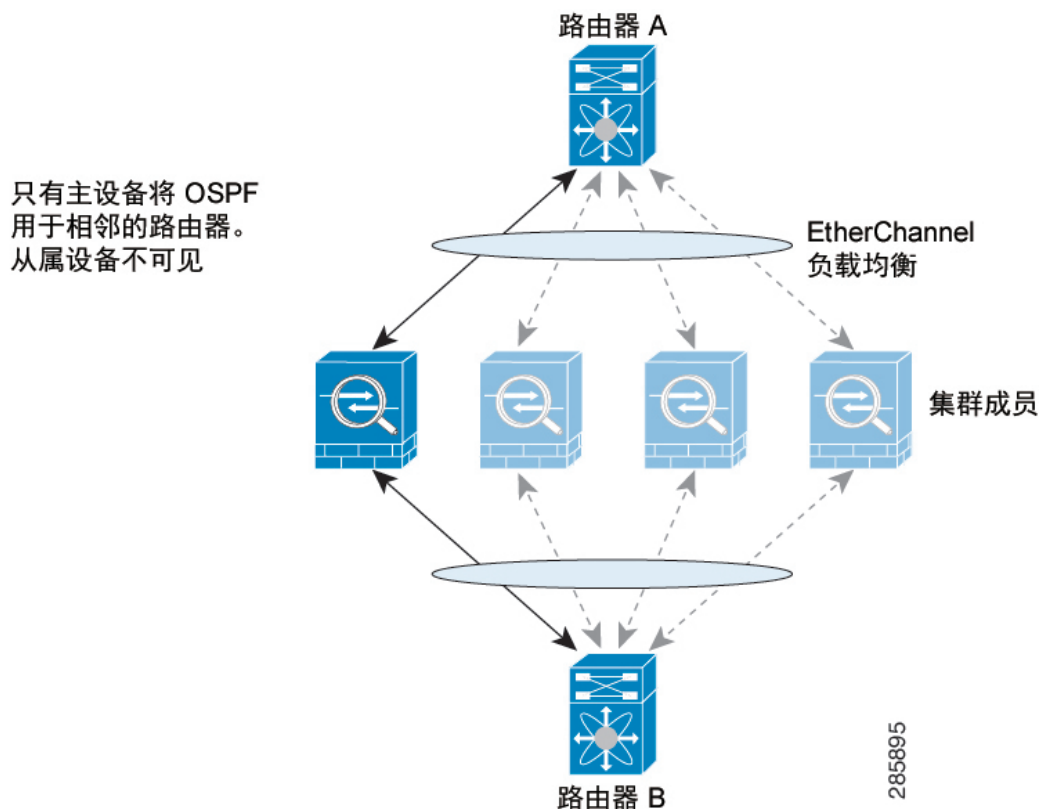
图 59: 跨网络 EtherChannel 模式下的动态路由
