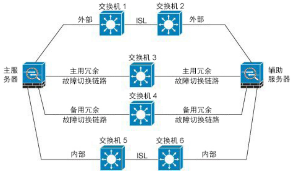
图 44: 使用交换机间链路连接
