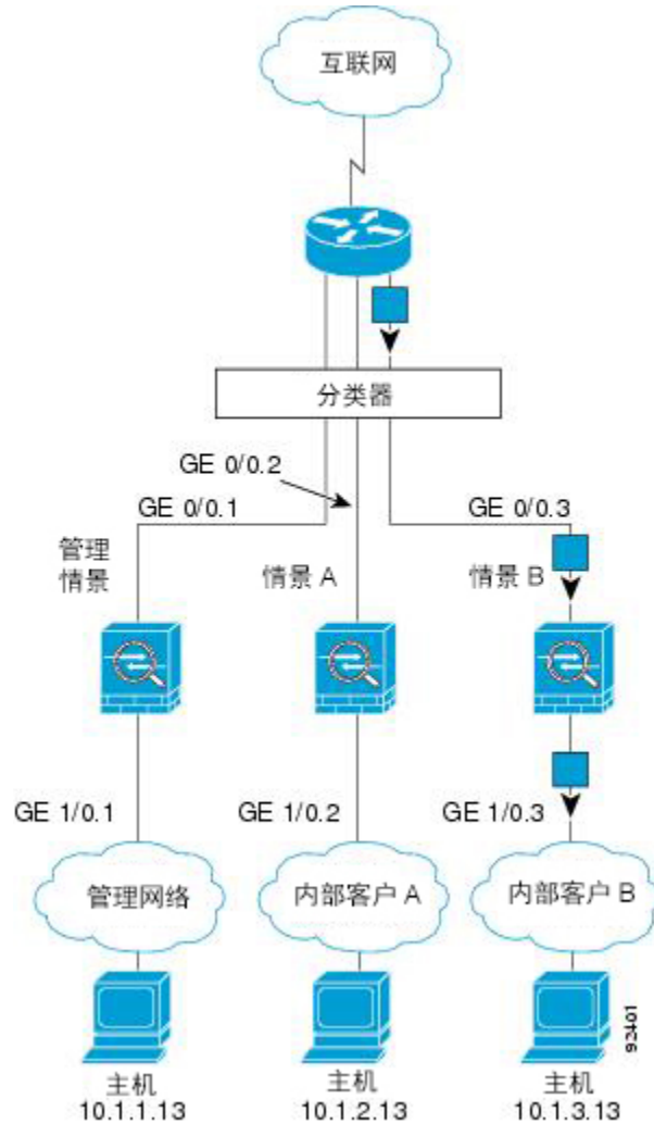
图 33: 透明防火墙情景
