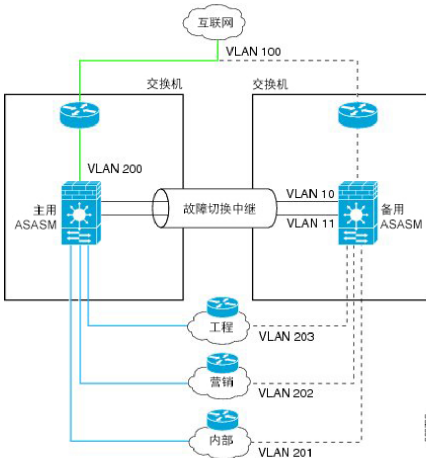
图 46: 正常运行
