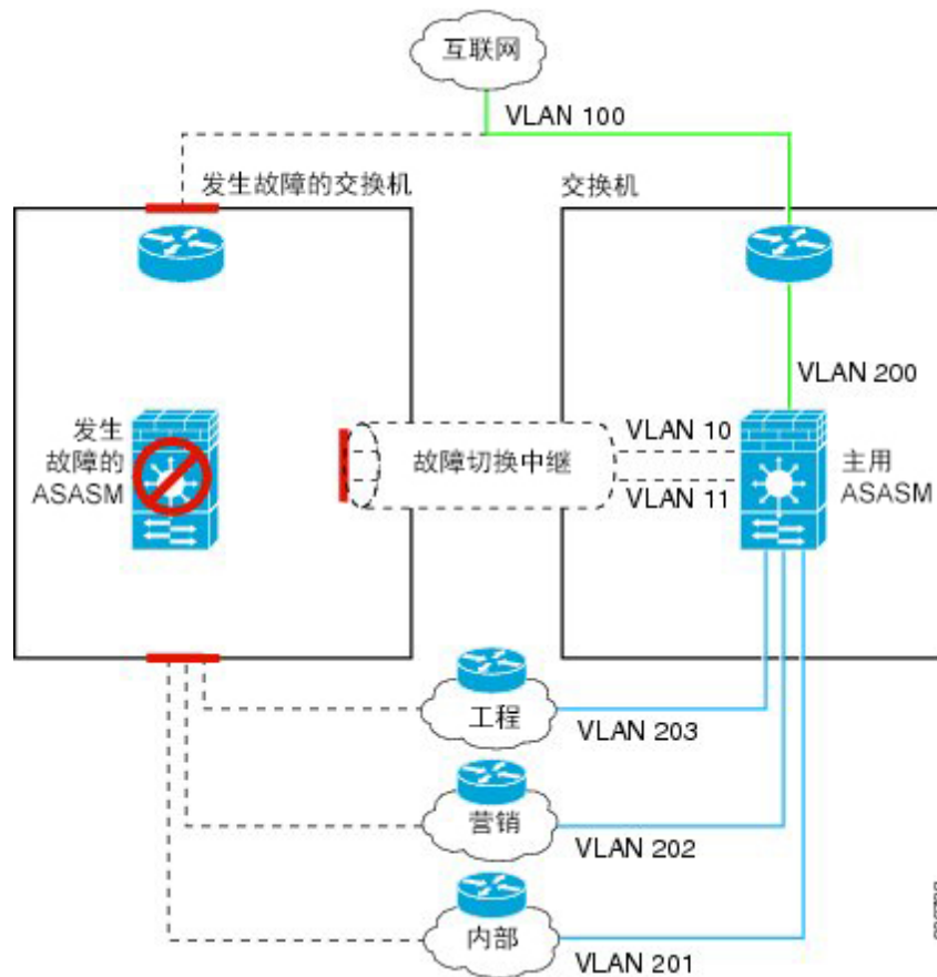
图 48: 交换机故障
