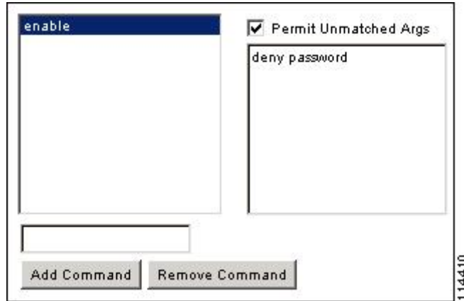
图 70: 禁止参数
