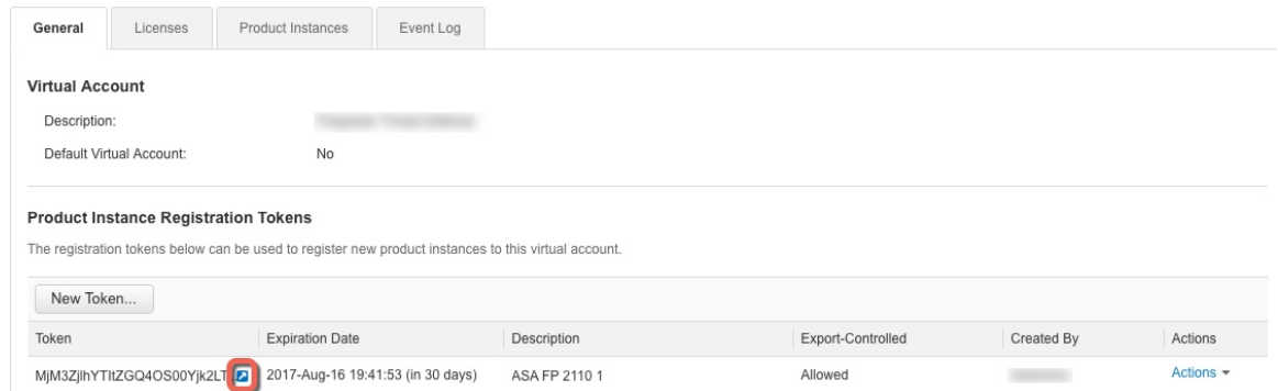
图 11: 复制令牌
