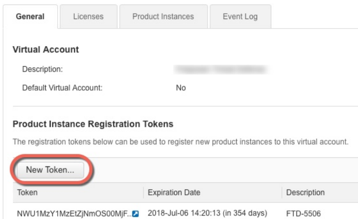
图 13: 新建令牌
