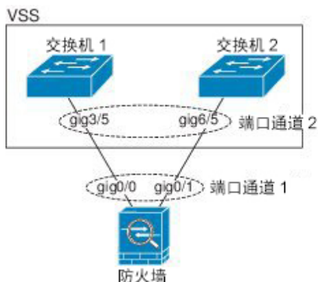
图 55: 连接至 VSS/vPC
