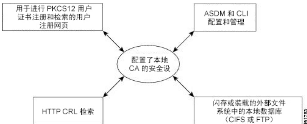
图 57: 本地 CA
