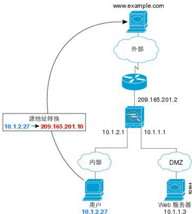
图 21: 内部至外部
