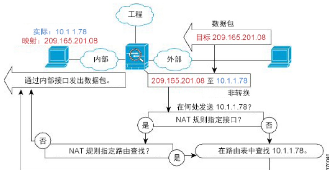
图 58: 含 NAT 的路由模式出口接口选择
