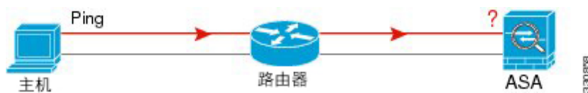
图 74: IP 寻址问题引发的 ping 故障
