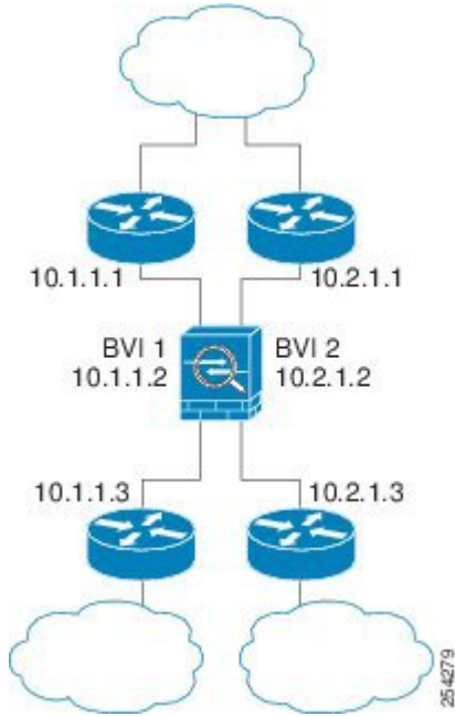
图 18: 具有两个网桥组的透明防火墙网络
