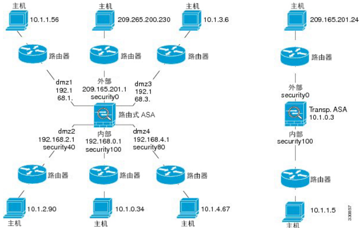
图 72: 接口、路由器和主机的网络图
