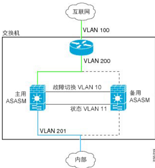
图 45: 交换机内故障切换
